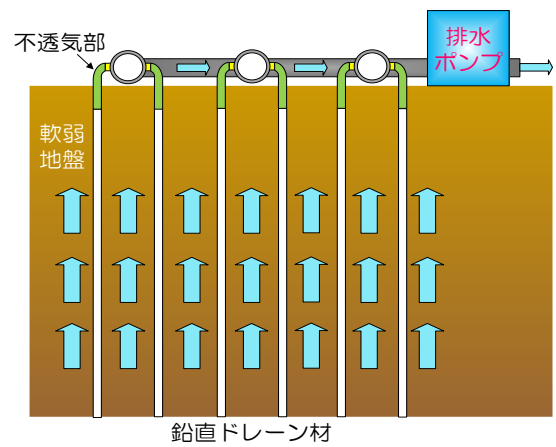
図-2 マルチサクシヨンドレーン断面図
