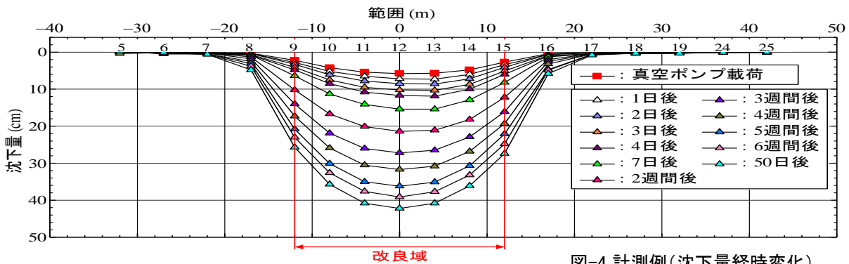
図-4 計測例(沈下量経時変化)
