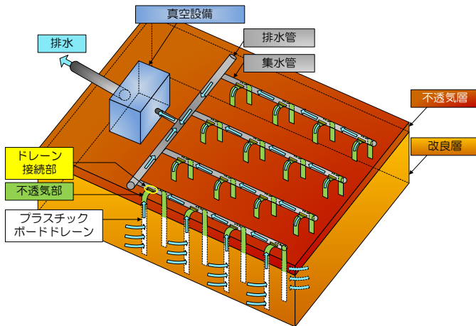
図-1 マルチサクシヨンドレーン概要図
