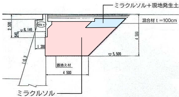
図-1 既設橋台背面での事例断面図
