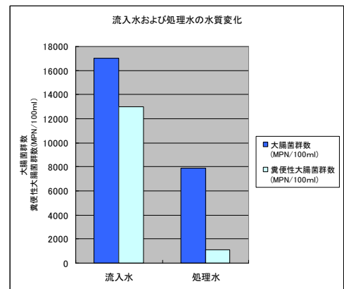
図-2 ダム流入河川浄化施設大腸菌郡数
