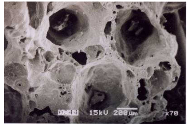
写真-2 ミラクルソル内部顕微鏡写真
