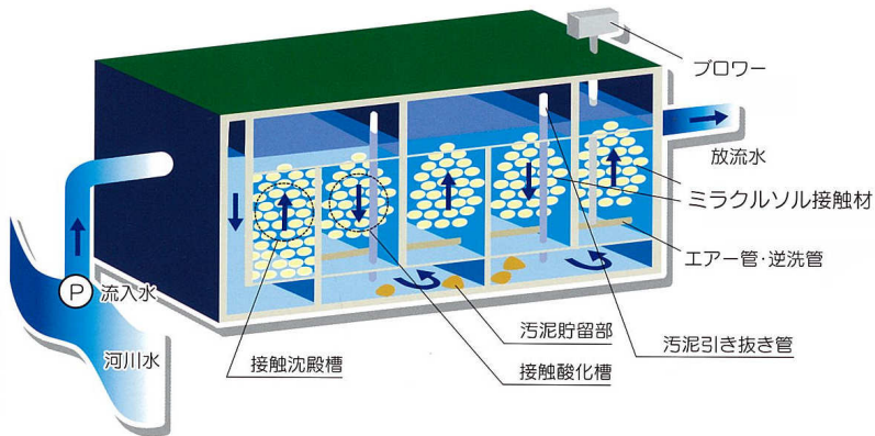
図-1 ミラクルソル水質浄化システム
