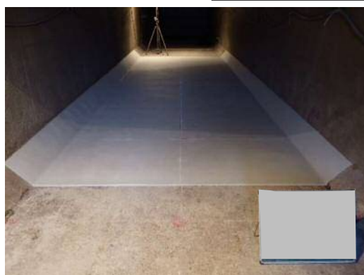
川島樋門（宮崎県）
