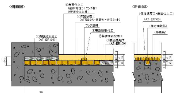
< AT-P工法施工断面図 底板部 >
