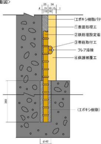
< AT-P工法施工断面図 柱壁部 >
