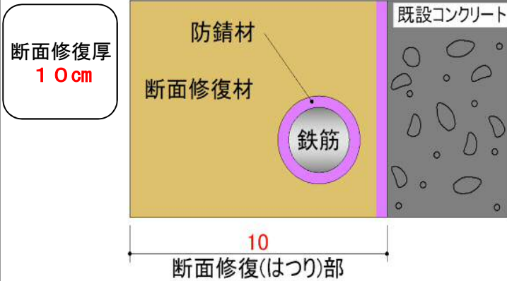
断面修復工施工断面図
