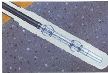
5. 緊張 グラウトが所定の強度に達した所で、緊張作業を行います。プレート背面防食のために、ストップパースを取付け、緊張力とアンカー頭部の変位を確認しながら緊張作業を行います。
