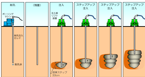
図-2 施工手順
