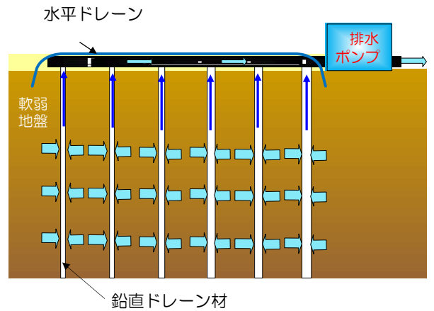
図-1.2 ジオドレーンSPD工法概念図
