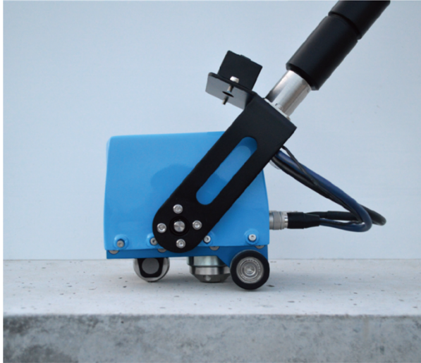
ブルードクター (電磁ハンマー体型センサユニット)
