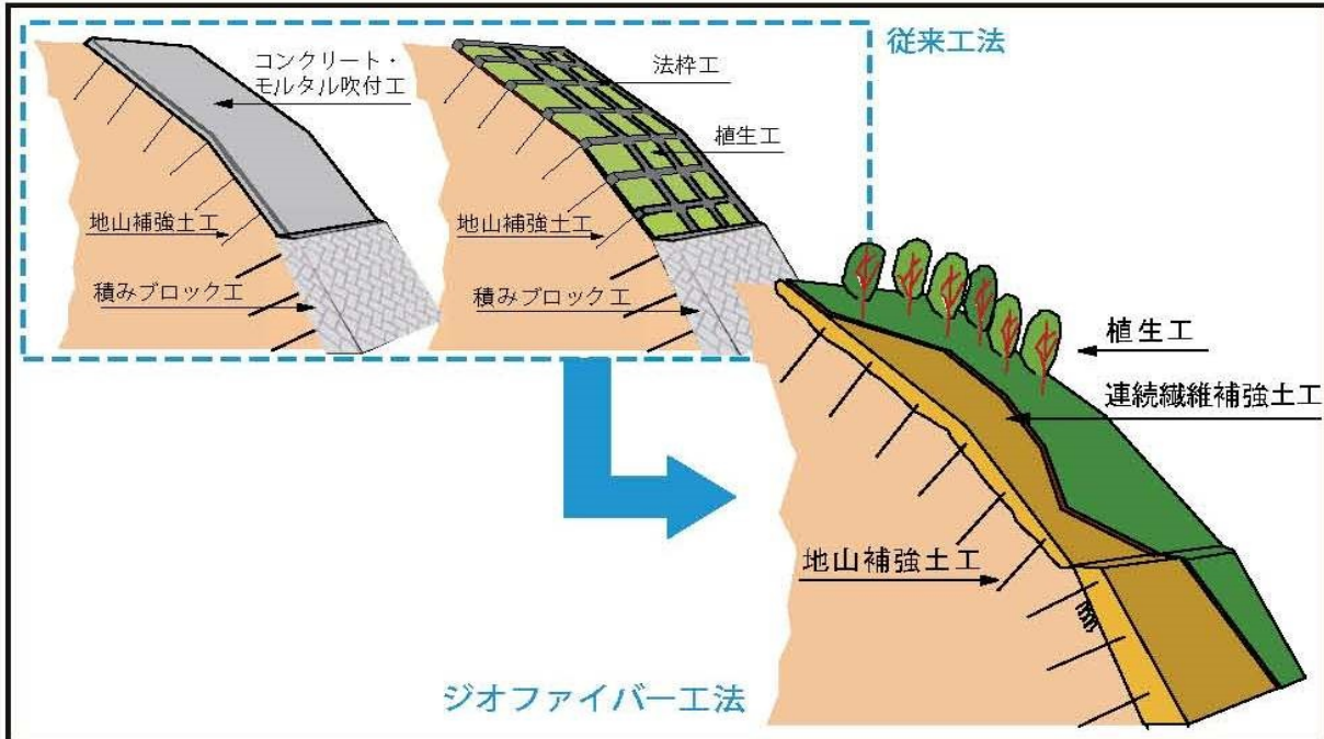
従来工法とジオファイバー工法の比較
