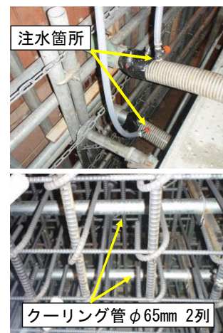
写真-3 クーリング状況
