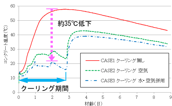
図-2 コンクリート温度履歴図
