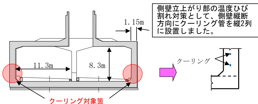
図-3 函渠構造物断面図
