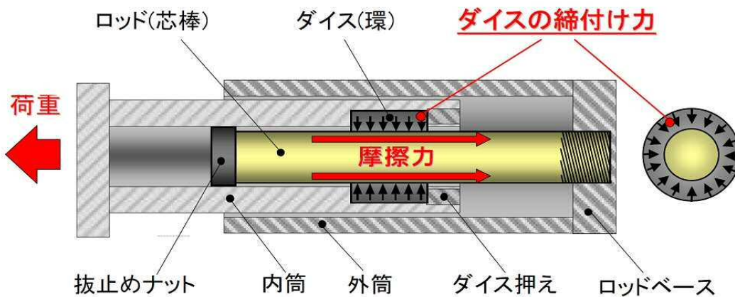
図-2 摩擦機構概要
