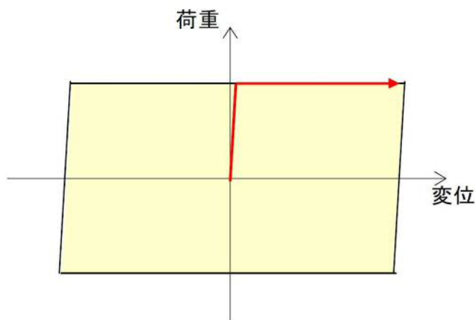
図-3 摩擦ダンパーの履歴特性
