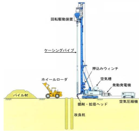
施工概要図
