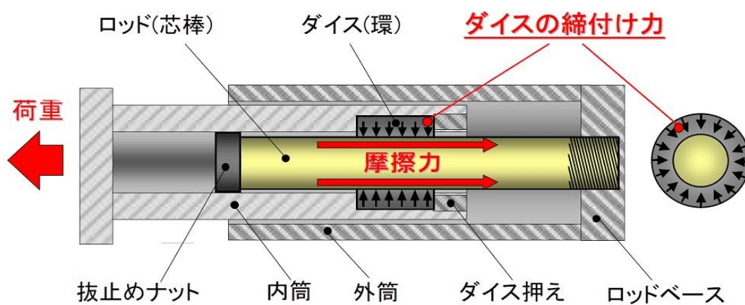
図-2 摩擦機構概要
