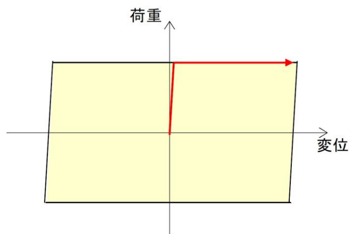
図-3 摩擦ダンパーの履歴特性
