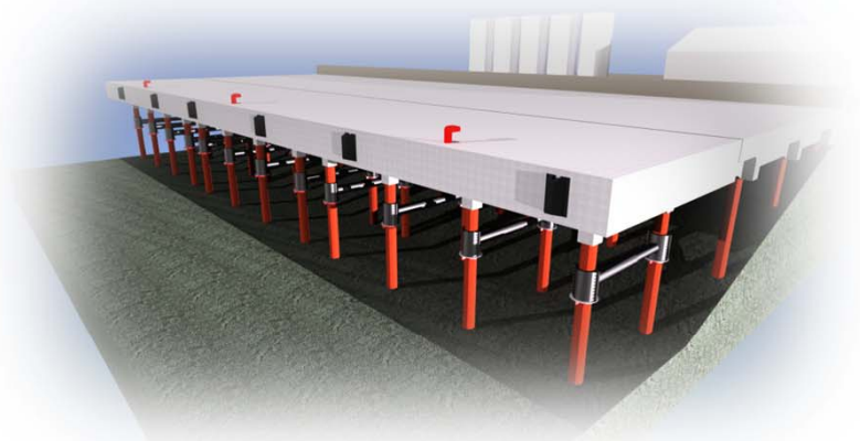
Re-Pier工法による耐震補強イメージ
