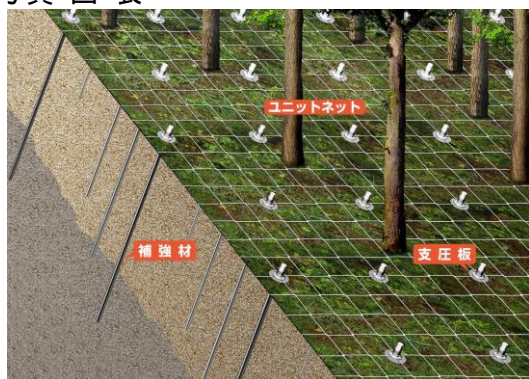
工法概略図
