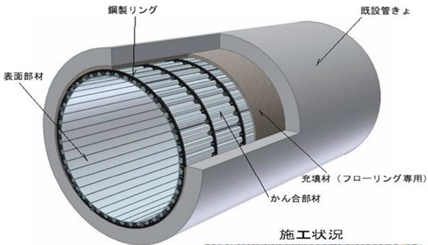
更生断面 詳細図
