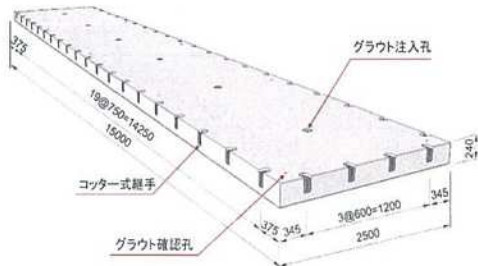
高強度PRC版 標準図 (重荷重用)
