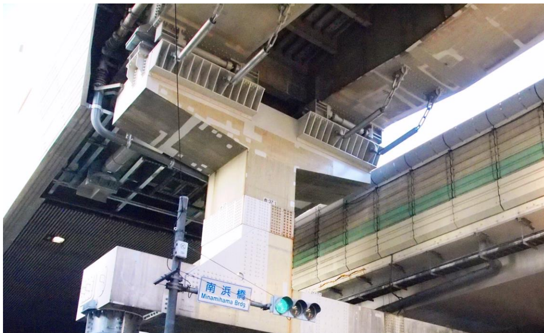
図-2 設置例
