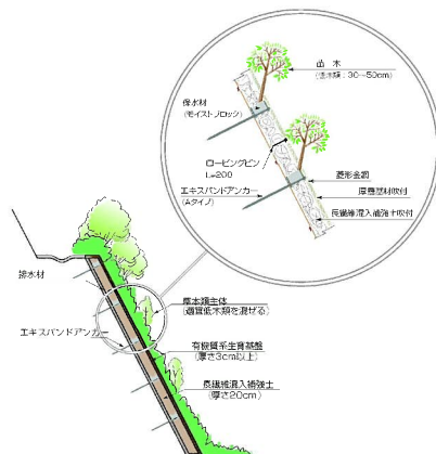
法面保護タイプ
