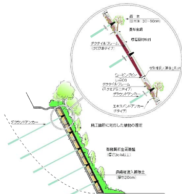
法面安定タイプ
