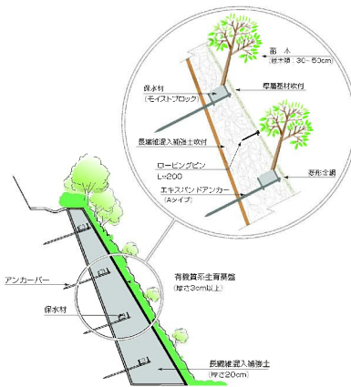
擁壁タイプ
