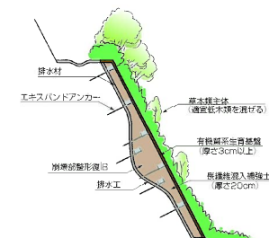
擁壁タイプ(崩壊部復旧タイプ)
