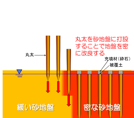
図-1 LP-LiC工法の液状化対策原理
