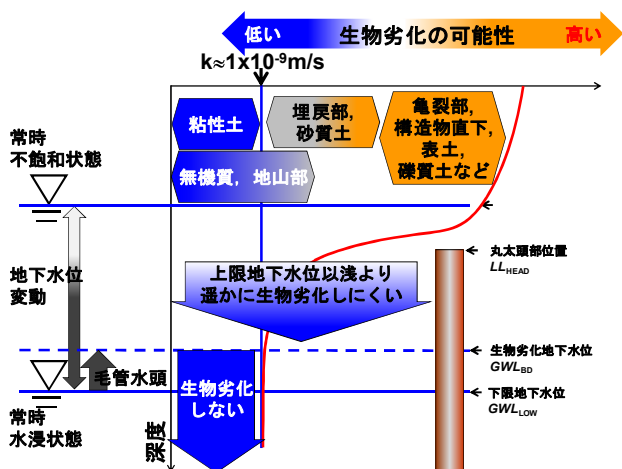
図-5 地中における木材の生物劣化の可能性
