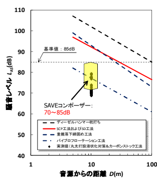
(b) 騒音レベル
