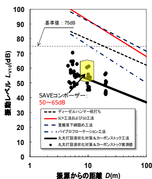
(a) 振動レベル
