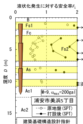
図-2 LP-LiC工法の液状化対策効果
