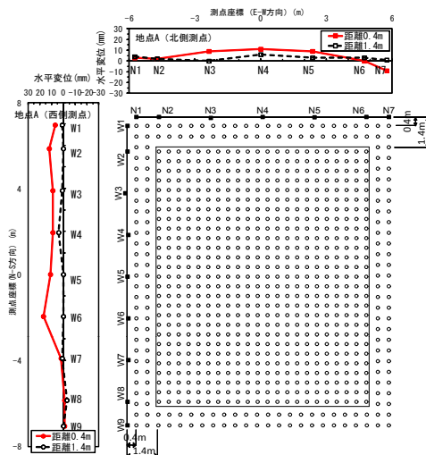
図-4 丸太打設による周辺地盤の変位
