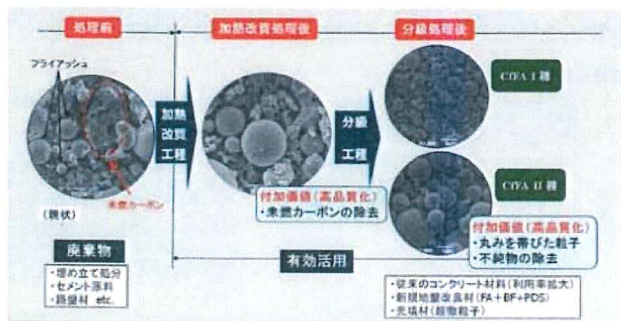
高品質フライアッシュの製造工程と電子顕微鏡（SEM）写真
