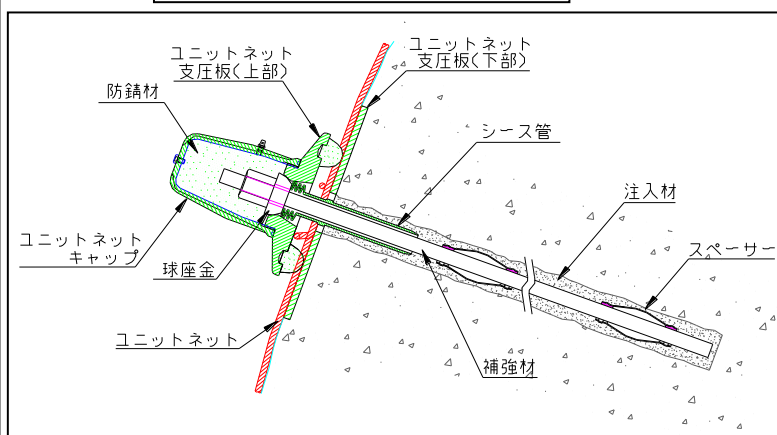
組み立て図
