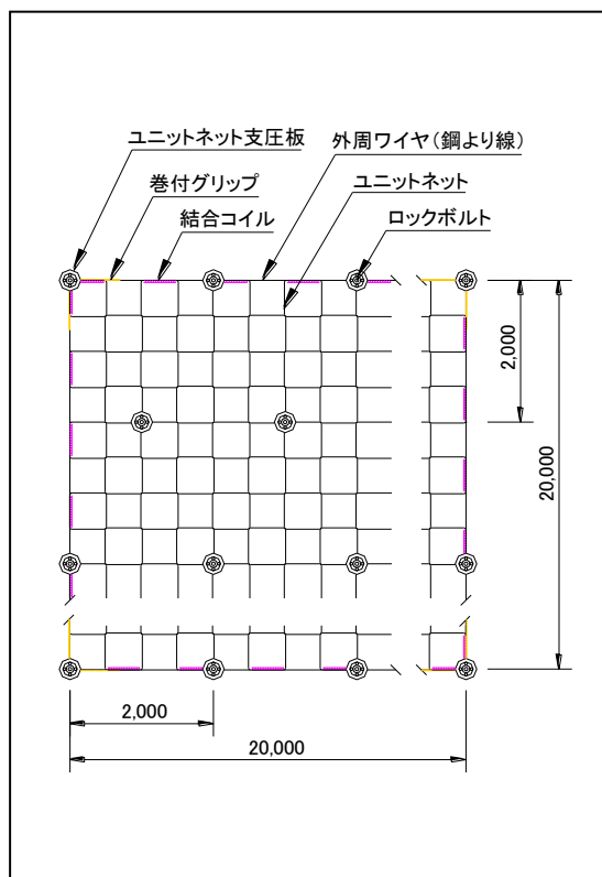
標準展開図
