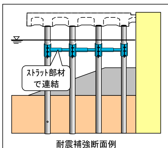
Re-Pier（伸縮式ストラット）工法による耐震補強イメージ
