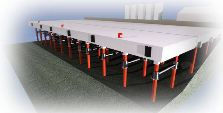
Re-Pier（伸縮式ストラット）工法による耐震補強イメージ
