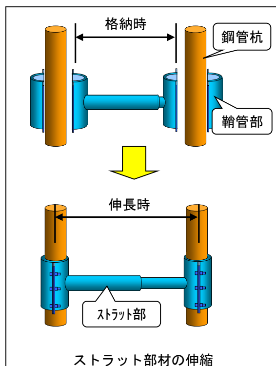
Re-Pier（伸縮式ストラット）工法による耐震補強イメージ
