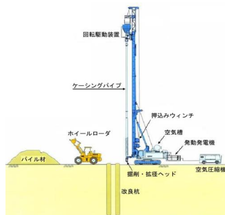
施工概要図
