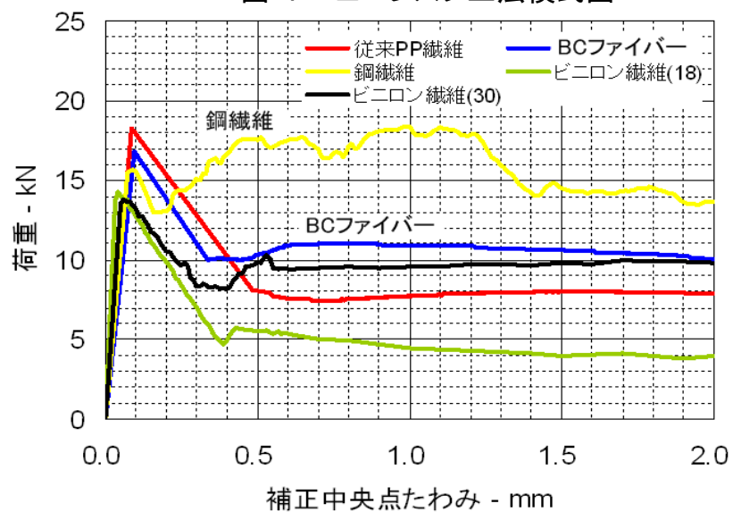
図-2 各種繊維補強モルタルの曲げタフネス試験
