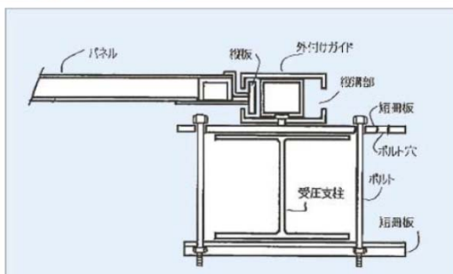
支柱に取り付けた詳細図
