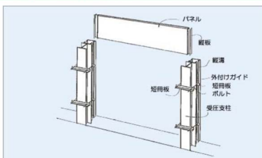
パネル式防護柵のイメージ
