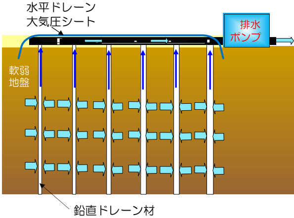
図-1.2 ジオドレーンSPD工法概念図
