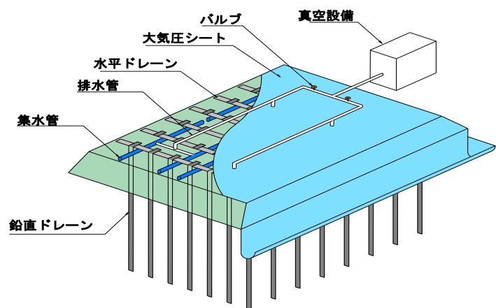
図-1.1 ジオドレーンSPD工法概要図
