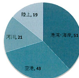
図-4 対象物ごとの施工実績(134件)
