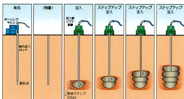
図-2 施工手順
