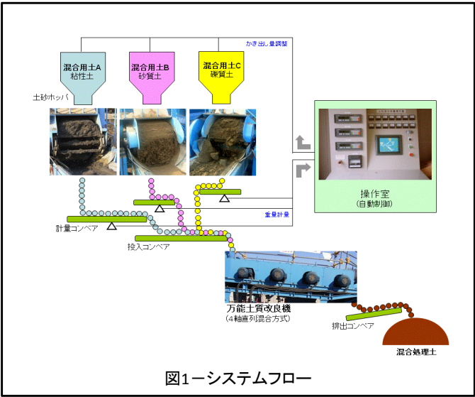
小竹町ストックヤード(A)土砂改良工での混合事例(3種混合)
