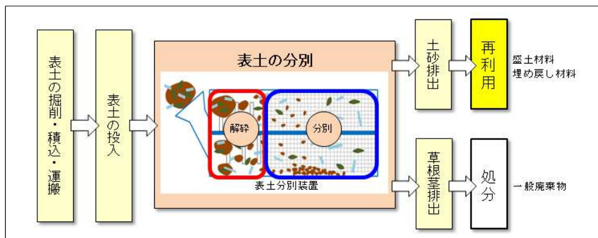
図1-土砂分別フロー
