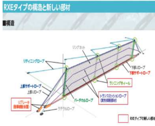
RX-Eシリーズ (500~30,00kJ)対応, 伸び量30~40%軽減
