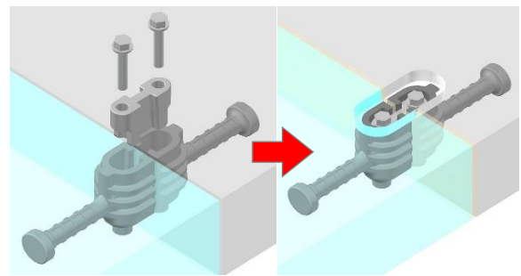
コッター式継手による連結イメージ
