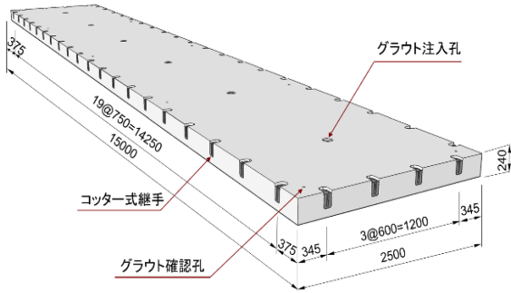
高強度PRC版 標準図 (重荷重用)
