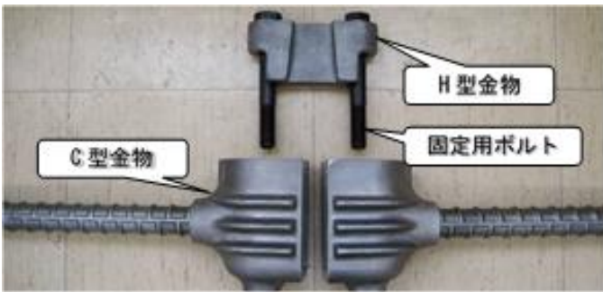
コッター式継手
