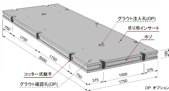
道路用PRC版 標準図
