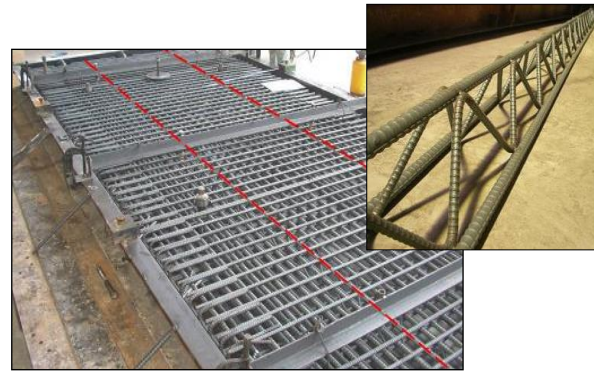
鉄筋籠(左)とラチストラス鉄筋(右)
