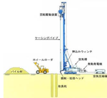
施工概要図
